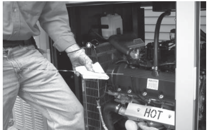
Figura 1.14 - Comprobación del aceite de motor
